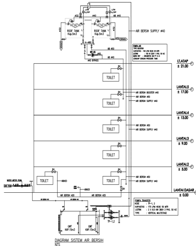
Gambar 5. Skematik Plambing Air Bersih Hotel
